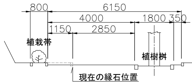
①-① 断面図
