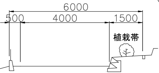
③-③ 断面図
