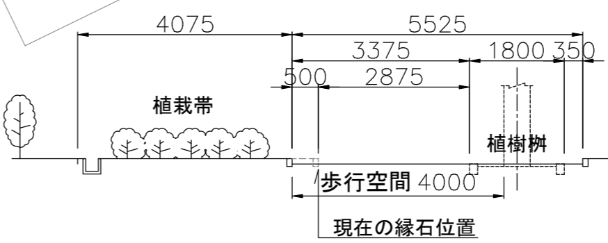
②-② 断面図
