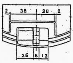
蓋蓋式安裝圖
