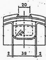
蓋蓋式F-1六角蓋圖
