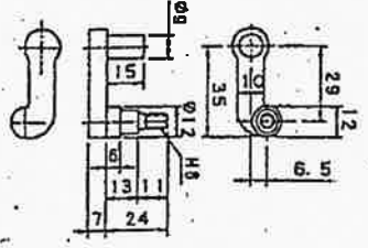
3 蓋蓋金飾螺絲
